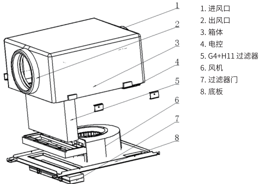
CF2-F200、CF2-F300 结构图
