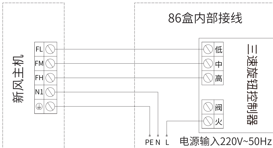
CF2-F200M~300M 三速旋钮控制器接线
