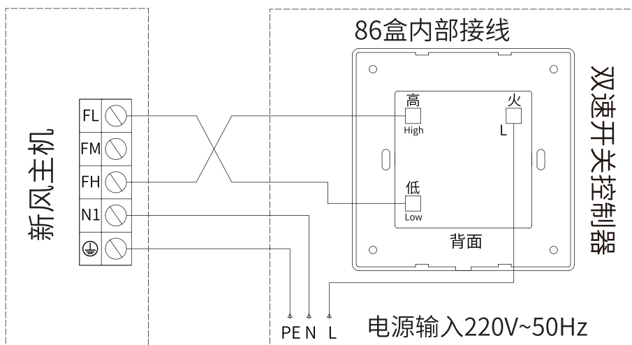
CF2-F200M~300M 双速开关控制器接线
