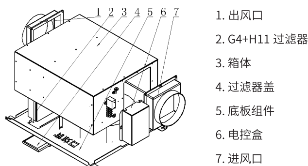
CF2-F200M、CF2-F220M、CF2-F300M 结构图
